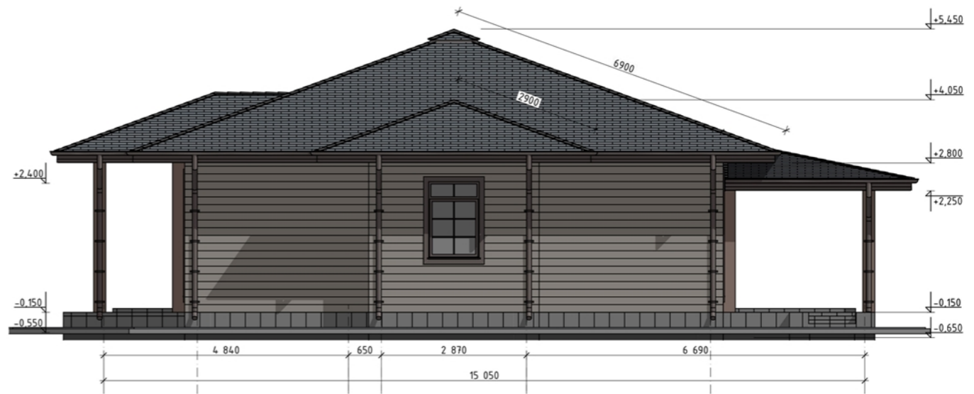
Фасад в осях (Ж-А) М1:50.
